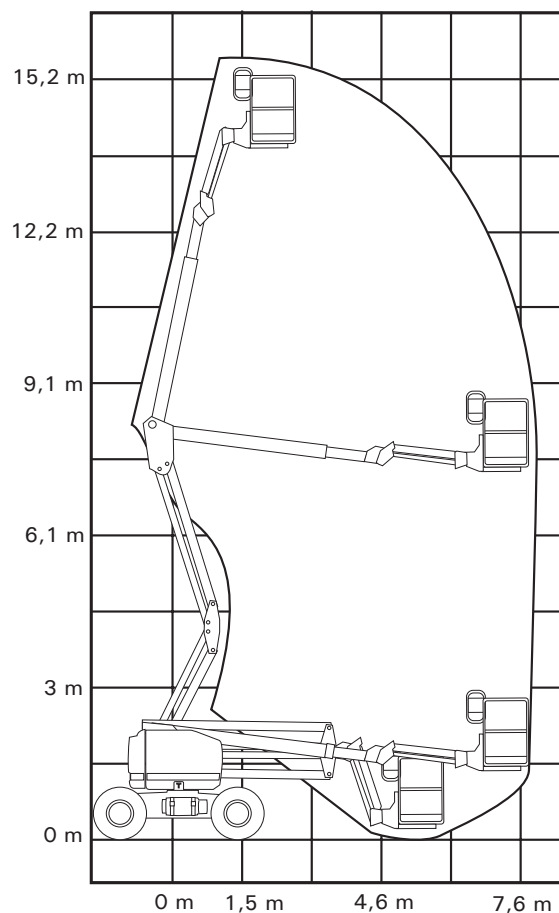
Werkbereik - modellen met jib
