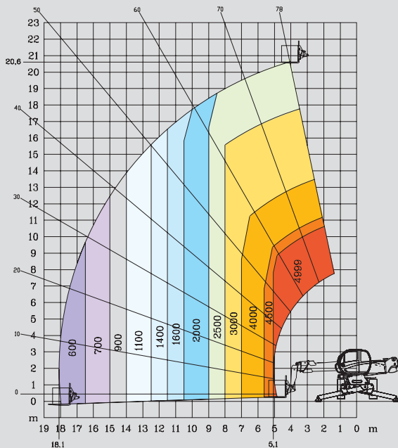
ROTATIE MET INGESCHOVEN STEMPELS MET VORKENBORD
