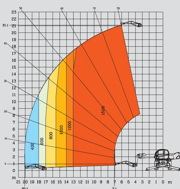
ROTATIE MET UITGESCHOVEN STEMPELS MET KRAANBALK P 1500
