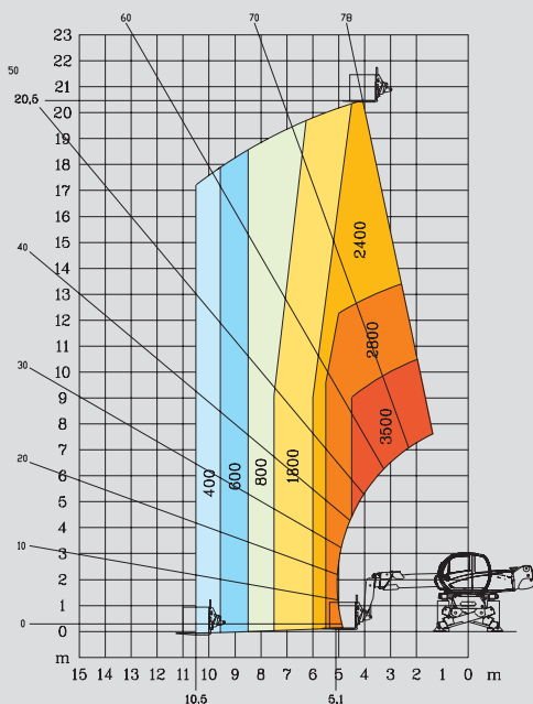
ROTATIE MET UITGESCHOVEN STEMPELS MET KRAANBALK P 600
