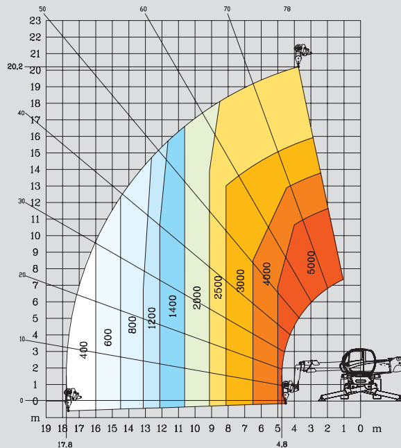
ROTATIE MET UITGESCHOVEN STEMPELS MET KRAANBALK P 1500
