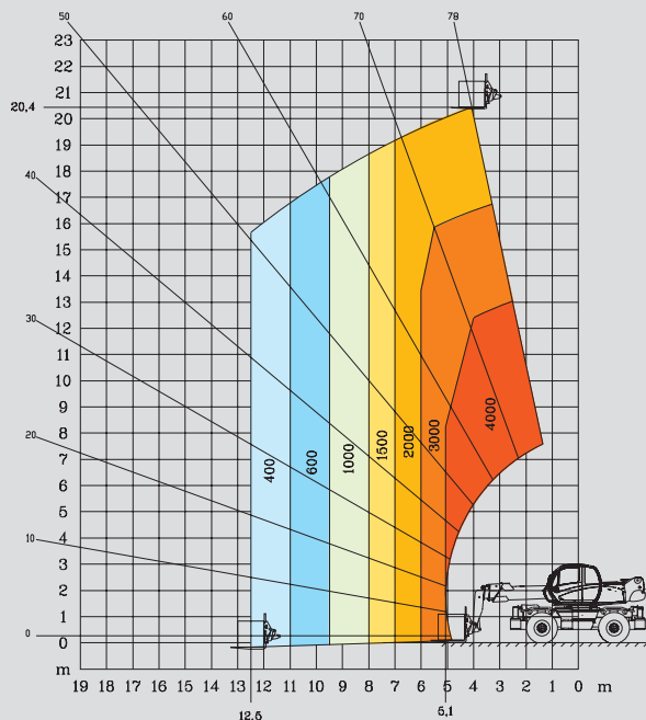
ROTATIE OP UITGESCHOVEN STEMPELS MET LIER 5 T
