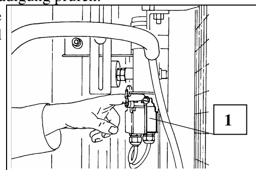
Fig. 51 Überlastendschalter
