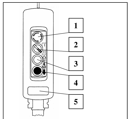
Fig. 8 Handsteuerung
