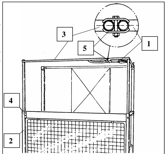
Fig. 19 Aufbau Spezialaufsteckrahmen
