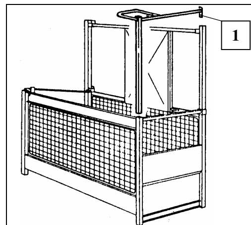
Fig. 16 Standardaufsteckrahmen
