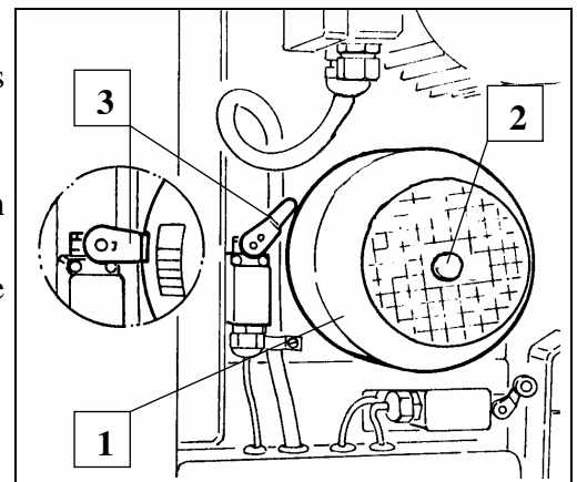
Fig. 50 Fangvorrichtung
