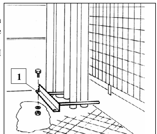
Fig. 20 Anbau Bodenrohrhalter
