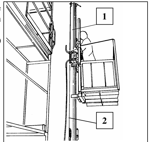
Fig. 28 Mast montieren
