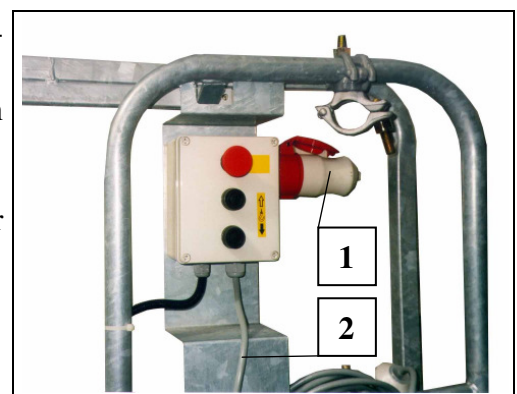
Fig. 45 Etagensteuerung einstecken
