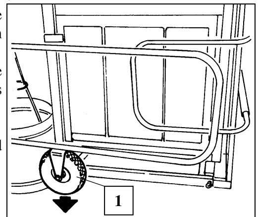
Fig. 24 Transporträder
