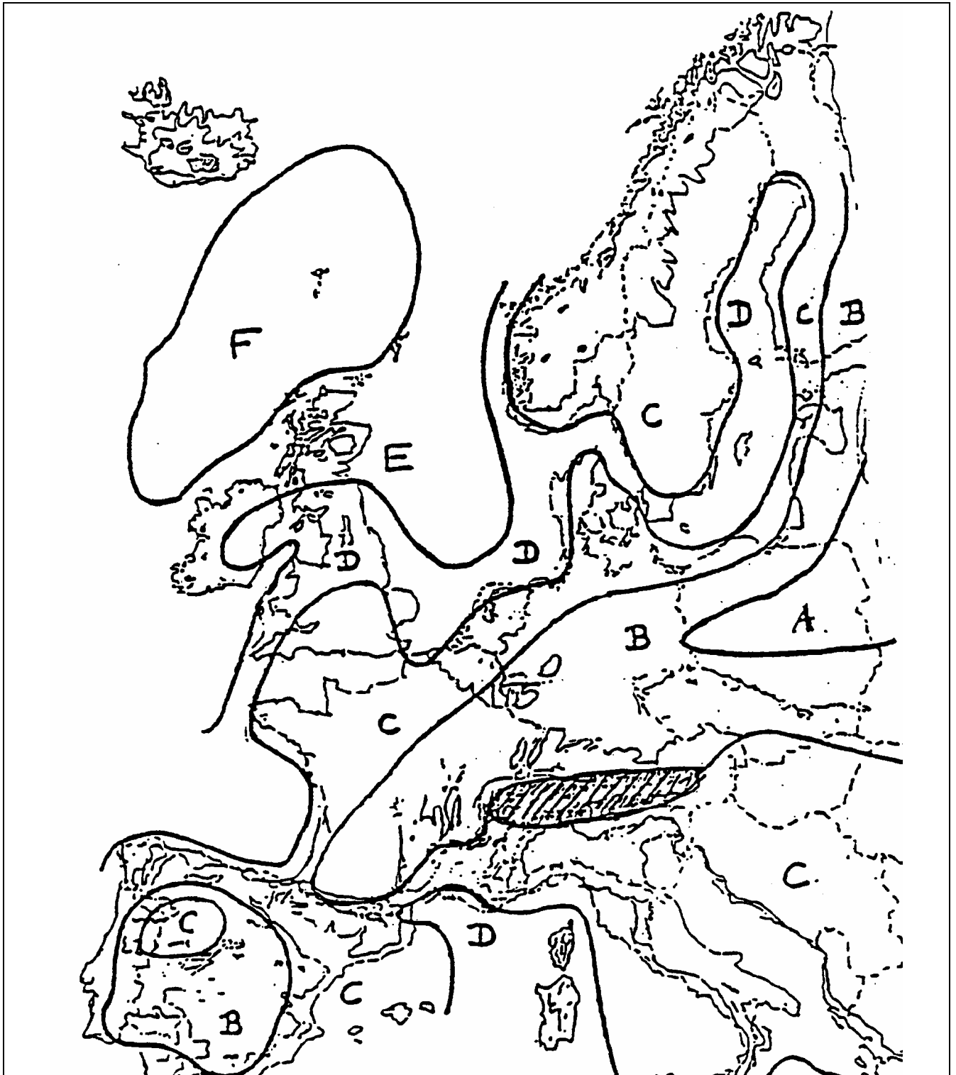
Fig. 37 Europäische Windkarte
