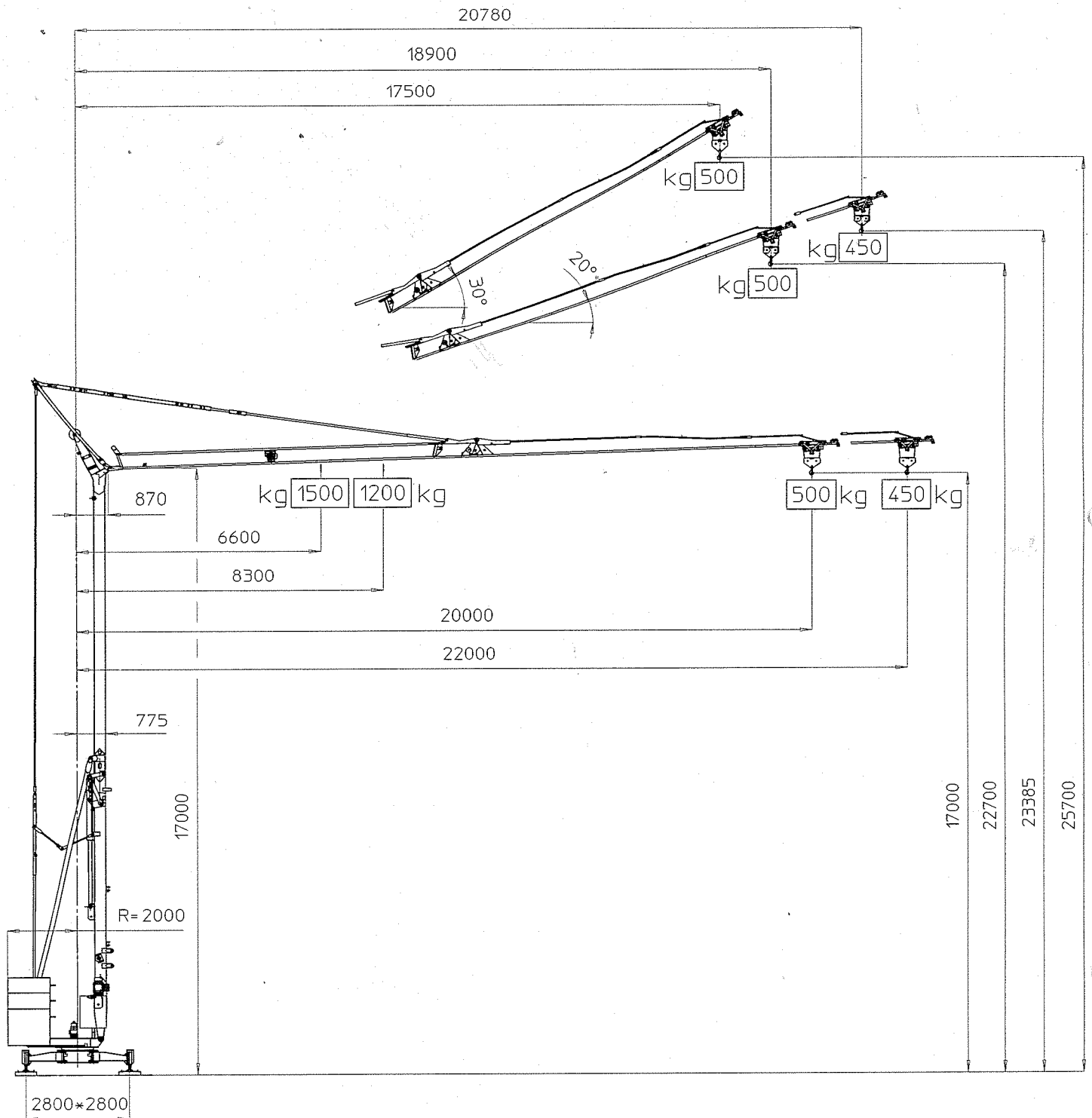
Schema van kraan OMV 168/22NL met arm van 20 m en vlucht tot 30° en arm van 22 m met vlucht tot 20°.
