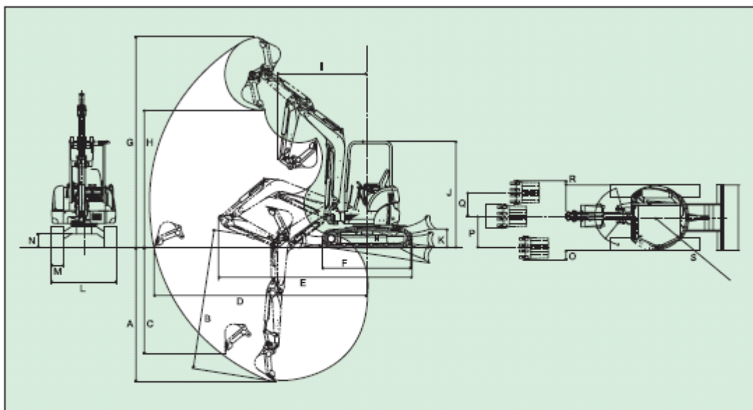
Dimensions
