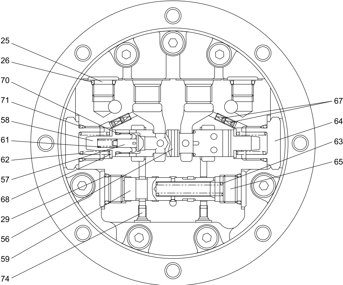
VIEW Y
