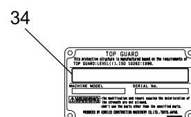
TOP GUARD 銘板 TOP GUARD PLATE 詳細 ee DETAIL ee 詳細 ff DETAIL ff
