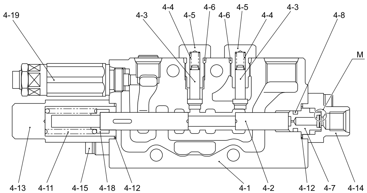
SECTION D-D
