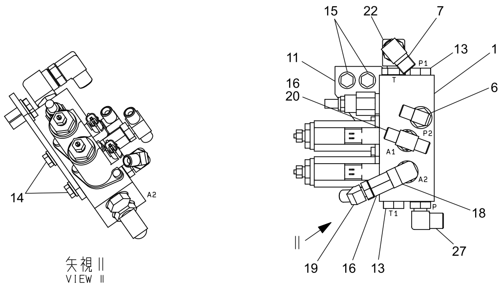
詳細 aa (ソレノイドバルブ詳細) DETAIL aa (DETAIL OF SOLENOID VALVE)
