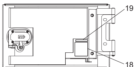
詳細 aa DETAIL aa パネル裏側を示す SHOW BACKSIDE OF PANEL
