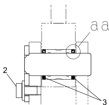
断面 A A SECTION AA
