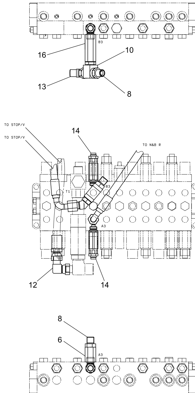
コネクタ取付詳細 DETAIL INSTALL CONNECTOR.
