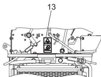
断面 CC SECTION CC
