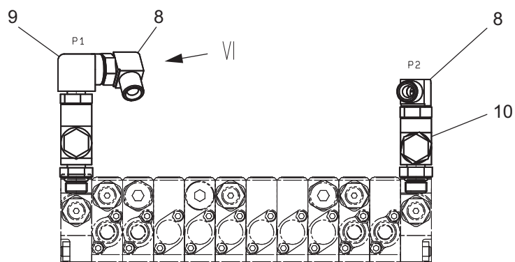
コネクタ取付詳細 DETAIL INSTAL CONNECTOR
