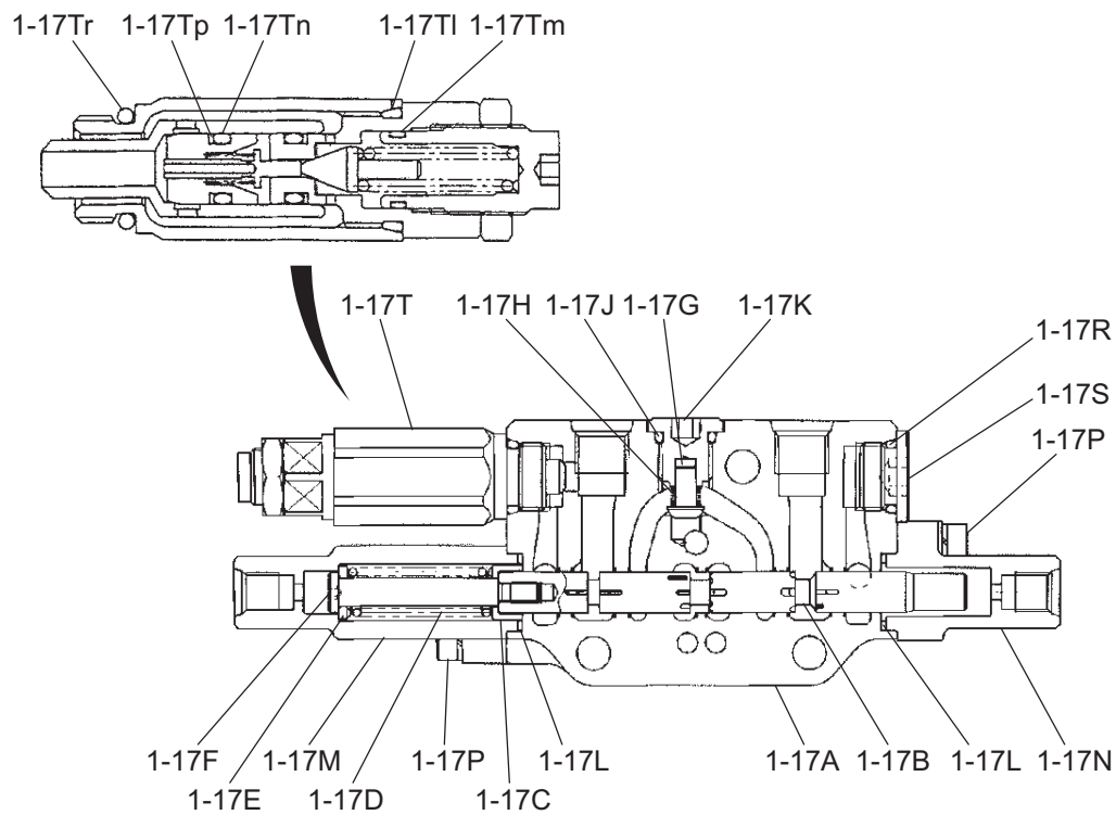
C-C (バケット・BUCKET)
