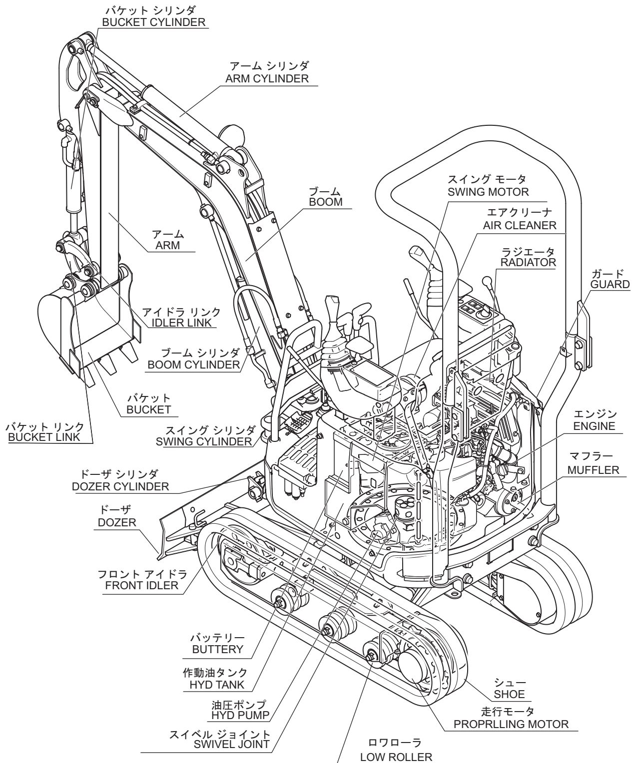
GENERAL DRAWING ・ 全体図
