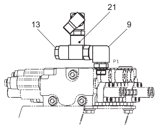
矢視 VI VIEW VI
