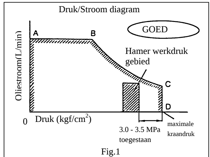
Voorbeeld van Druk/Stroom curve
