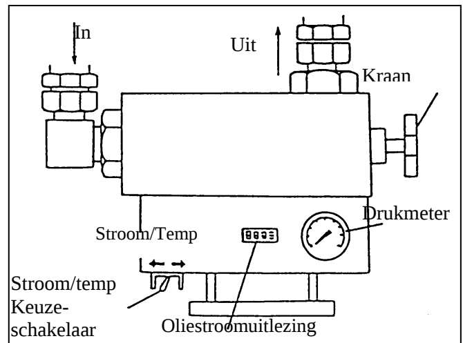
Typische oliestroommeter uitgerust met smoorventiel
