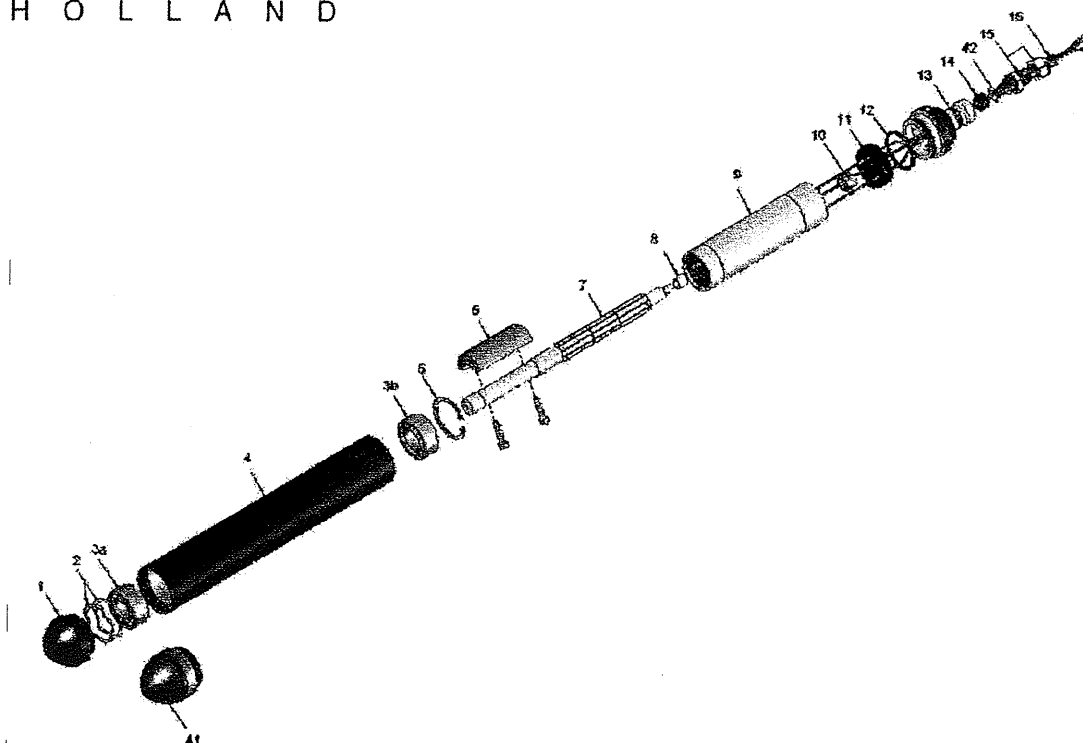
Figuur 4: Exploded view LHF-E trilfles korte uitvoering
