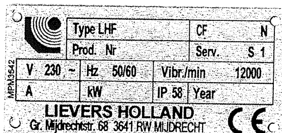
Figuur 1: Voorbeeld typeplaatje LHF-E
